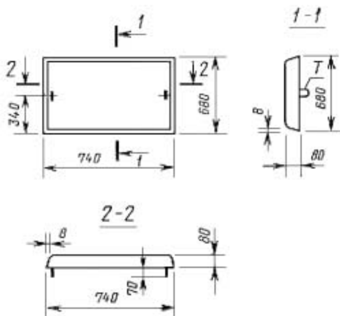
T - подъемная технологическая петля Черт. 3
