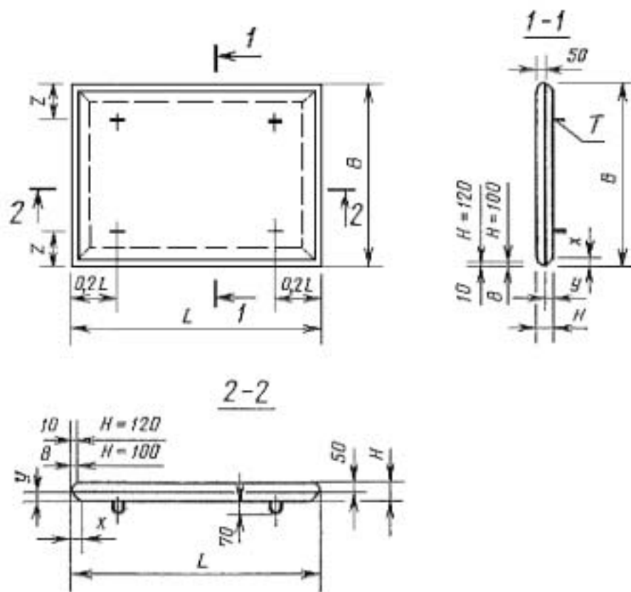
T - подъемная технологическая петля Черт. 2
