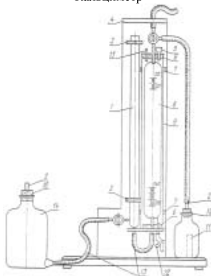
Кальциметр
