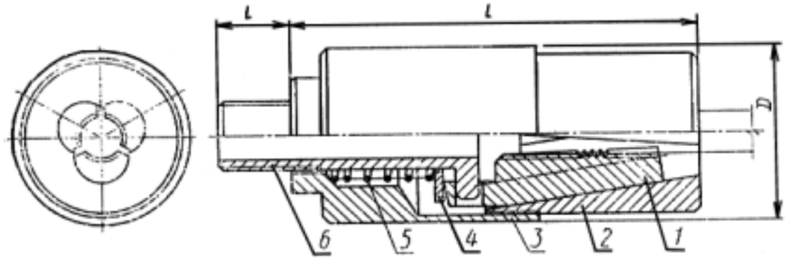
Зажим типа 1
