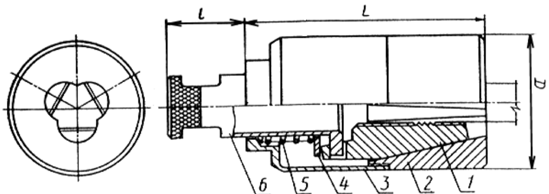
Зажим типа 3
