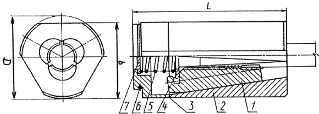
Зажим типа 2
