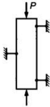
Рисунок 13 - Схемы закрепления стоек при испытании
