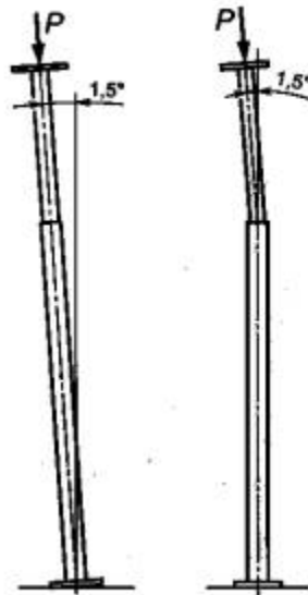
Рисунок 14 - Схема испытания составных стоек
