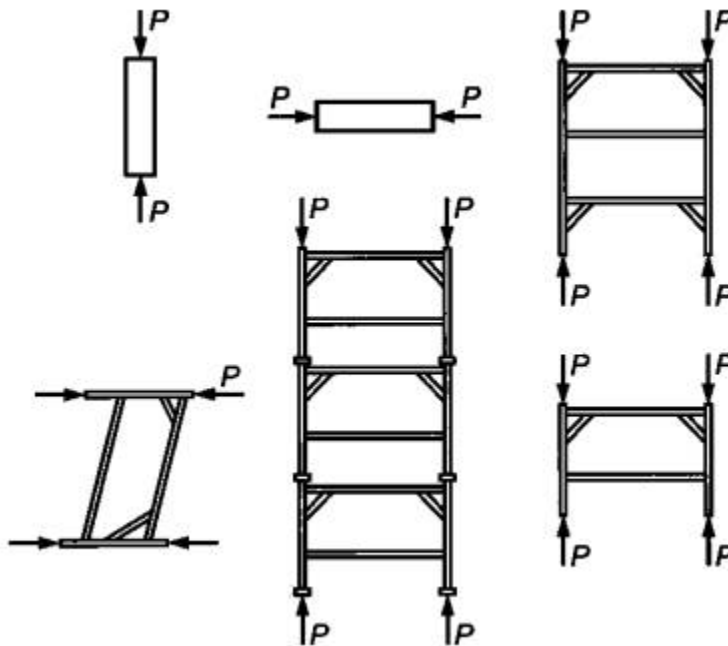
Рисунок 12 - Схемы испытания рам
