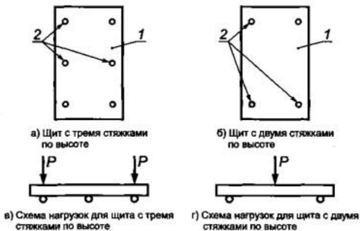
Рисунок 9 - Схема опор
